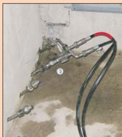
Injektionsdüsen werden in die Bohrlöcher eingesetzt.
